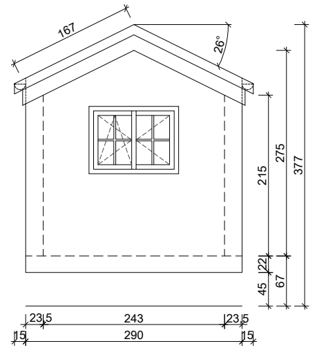
Ansicht D
