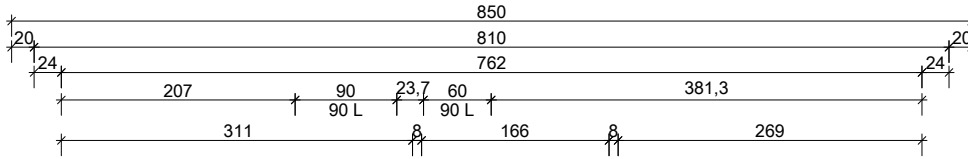
Ansicht A
